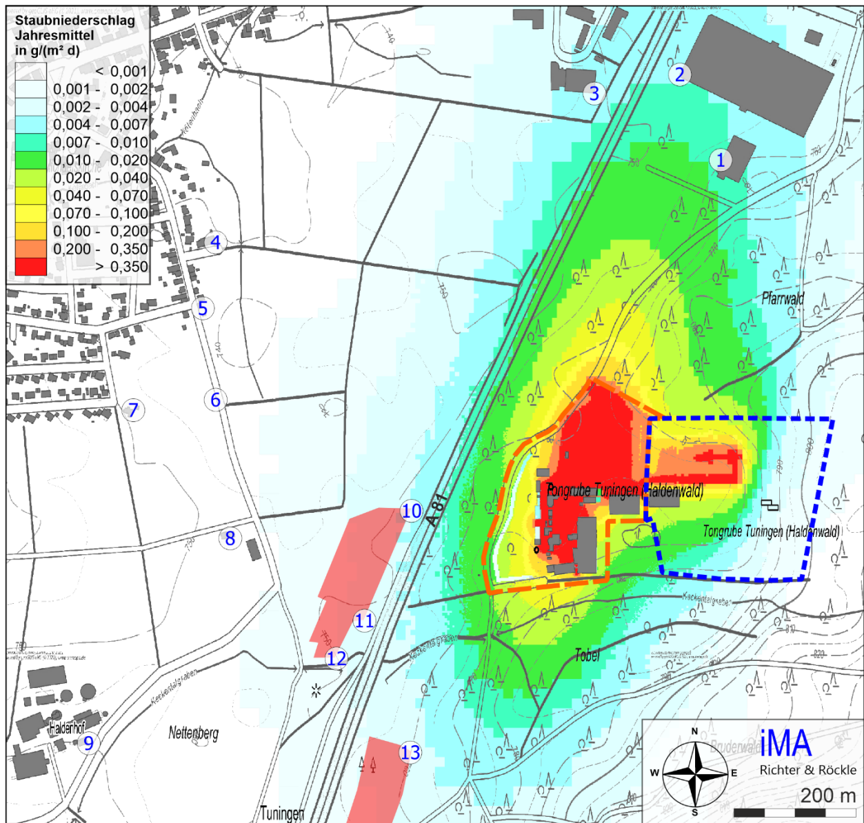
Abbildung A1-3: Staubniederschlags-Immissionsbeitrag der geplanten Anlagen.
