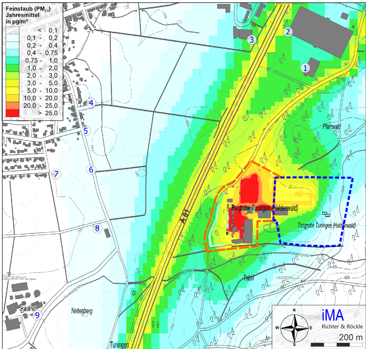
Abbildung A1-5: PM 2,5 -Immissionsbeitrag der geplanten Anlagen einschließlich des Beitrags der nahe gelegenen Quellen (siehe Kapitel 8.4.3 bis 8.4.5).
